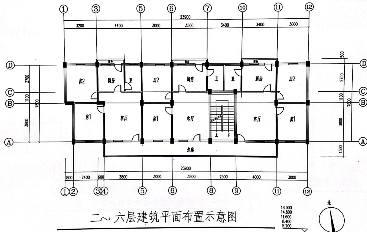
附件1：房屋建筑平面布置示意图（三）
