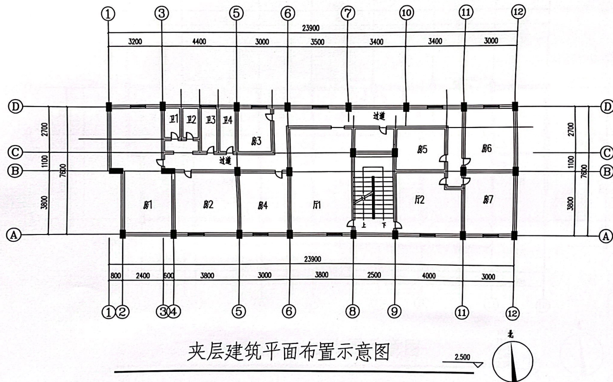
附件1：房屋建筑平面布置示意图（二）
