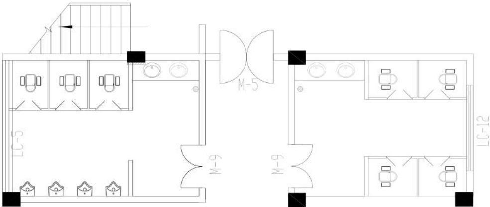
首层北面公卫原始图
