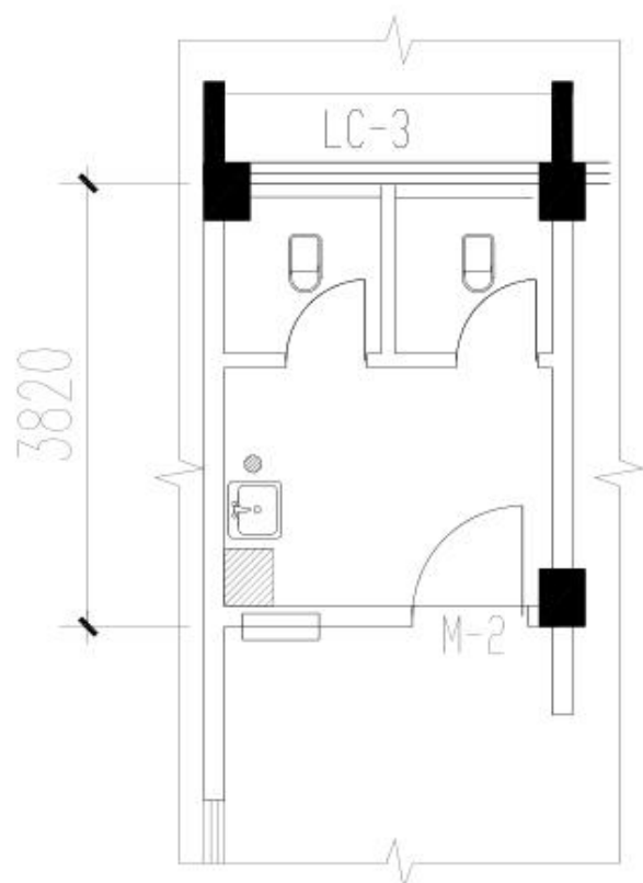
三层耳鼻喉科公卫原始图
