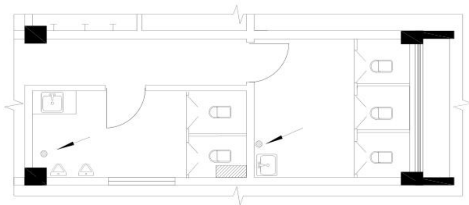
二层皮肤科公卫原始图
