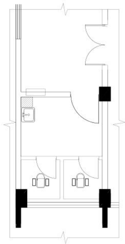
三层妇产科公卫1原始图
