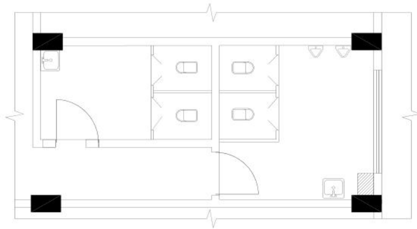
首层急诊公卫原始图
