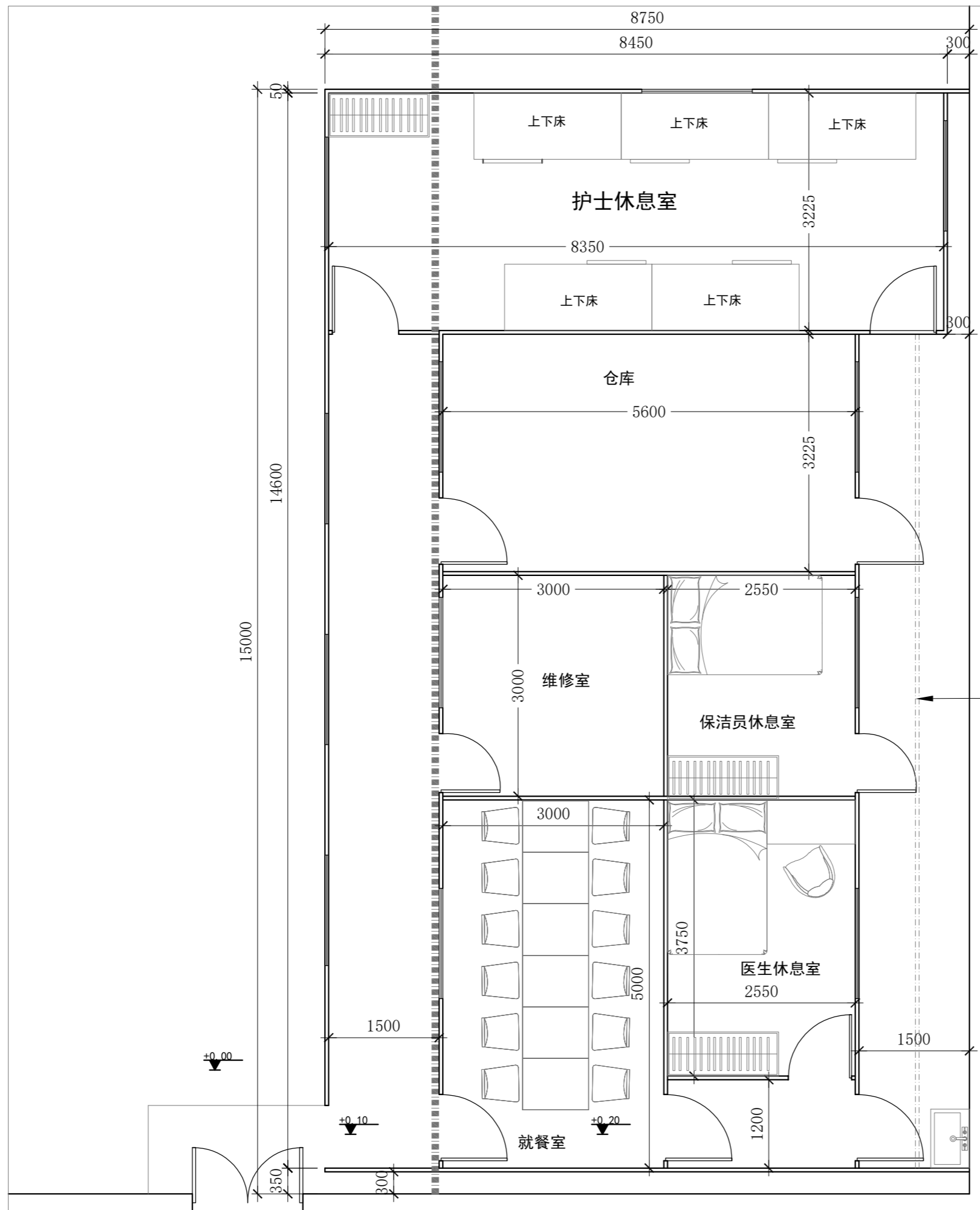
顺德区第三人民医院血透析休息室平面示意
